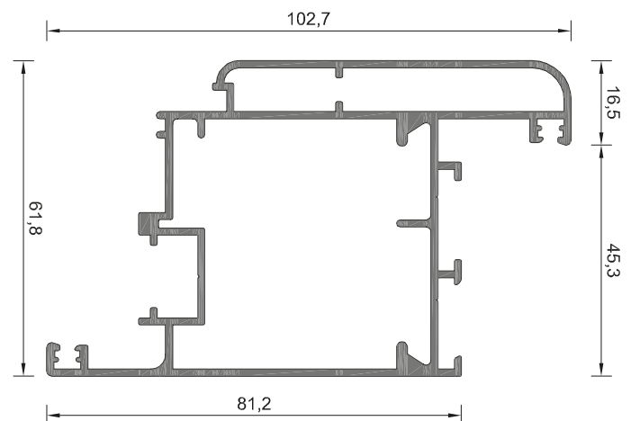
101-151 ΒΑΡΟΣ / WEIGHT 1651 gr/m
