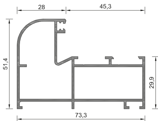
101-108 ΒΑΡΟΣ / WEIGHT 1100 gr/m
