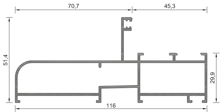
101-147 ΒΑΡΟΣ / WEIGHT 1226 gr/m
