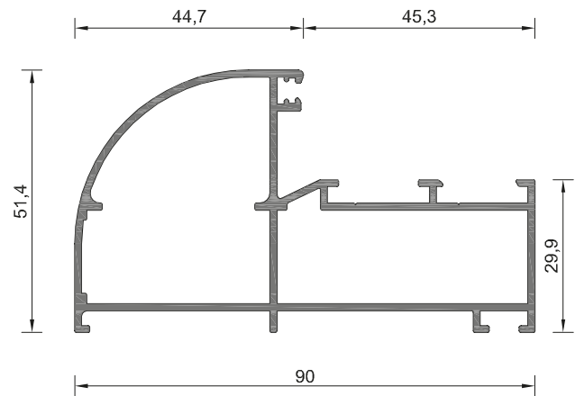
101-147 ΒΑΡΟΣ / WEIGHT 1226 gr/m
