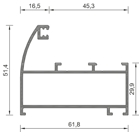
101-140 ΒΑΡΟΣ / WEIGHT 887 gr/m
