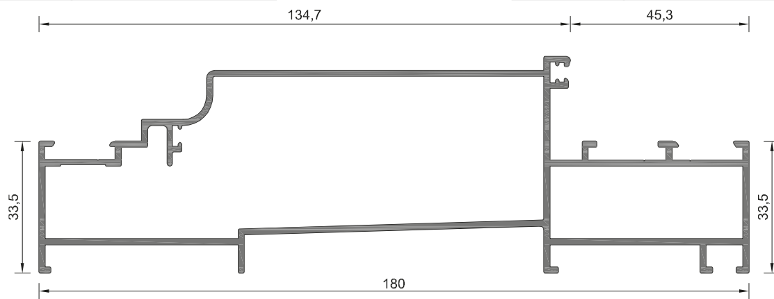
101-164 ΒΑΡΟΣ / WEIGHT 2263 gr/m
