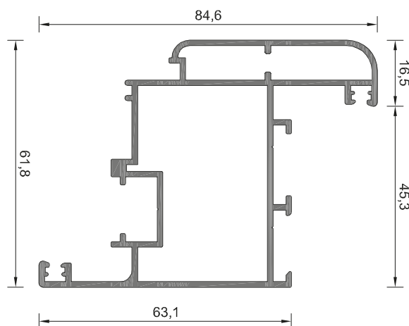
101-132 ΒΑΡΟΣ / WEIGHT 1326 gr/m
