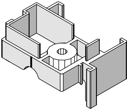
94-20-00-4205 ΤΑΠΑ ΓΙΑ ΜΠΙΝΙ ΦΙΛΗΤΟΥ 235-13 Rabbet seal plug for 235-13
