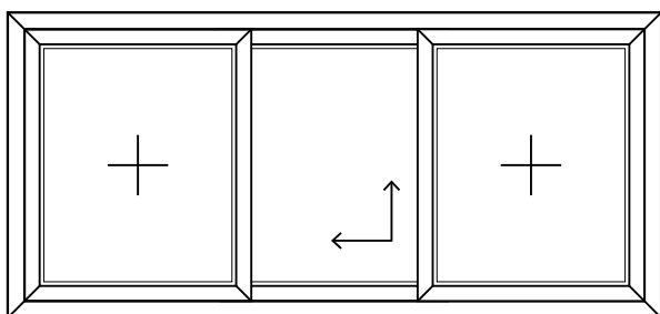
ΠΑΡΑΘΥΡΟ ΜΕ ΔΥΟ ΣΤΑΘΕΡΑ ΚΑΙ ΕΝΑ ΚΙΝΗΤΟ ΦΥΛΛΟ TWO FIXED AND A SLIDING WINDOW
