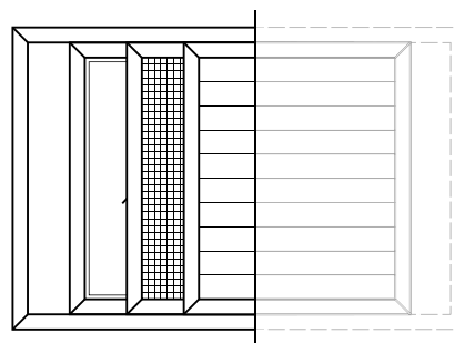
ΠΑΡΑΘΥΡΟ ΧΩΝΕΥΤΟ ΜΕ ΣΗΤΑ ΚΑΙ ΠΑΝΤΖΟΥΡΙ BUILD-IN WINDOW WITH MOSQUITO NET & SHUTTER
