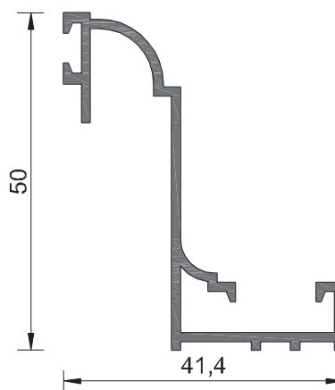
ΑΡΜΟΚΑΛΥΠΤΡΟ ΓΙΑ ΧΩΝΕΥΤΑ Cover gap for built-in window
