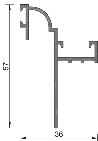
ΑΡΜΟΚΑΛΥΠΤΡΟ ΓΙΑ ΕΞΩΤΕΡΙΚΑ ΣΥΡΟΜΕΝΑ Cover gap for external sliding window
